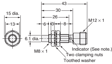
Fig. 18 : E2E-X4MD□-M1(G) E2E-X2ME□-M1/F□-M1
