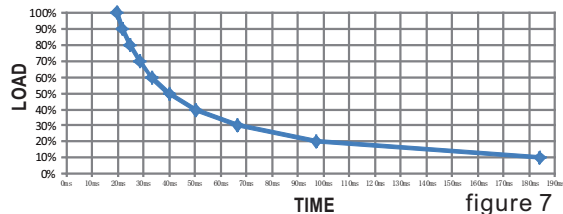
DDR-480D-48
