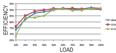
DDR-120C-24
