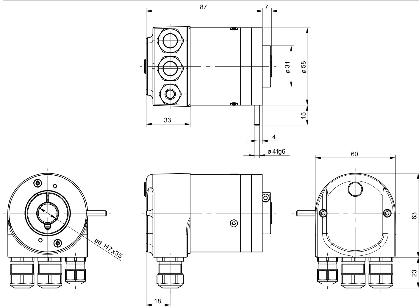
EN580C.ML-B - presse-étoupe, option MTQ003: pîge anti-rotation
