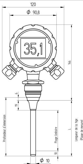
Raccord process en bas avec écrou-raccord, G 1 A hygiénique (BCID : A04), longueur de 200 mm ... 3000 mm
